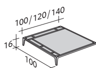
NON AUTOPORTANTE
