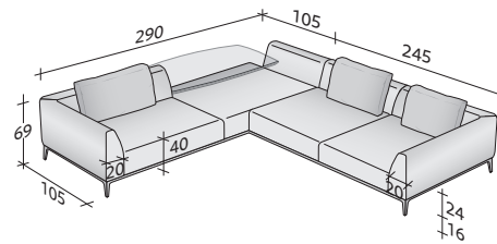
COMPOSIZIONE F (escluso tavolino)
