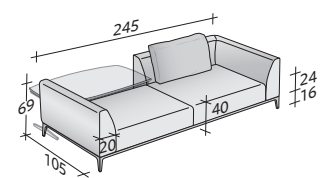
COMPOSIZIONE L (escluso tavolino)
