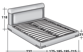
GESTELL H25 FESTE FEDERLEISTEN MIT HÄRTEREGULIERUNG ELEKTRISCH VERSTELLBARE FEDERHOLZRAHMEN
