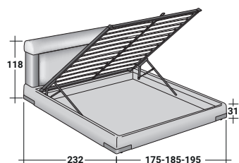
BETTKASTEN-GESTELL FESTE FEDERLEISTEN MIT HÄRTEREGULIERUNG
