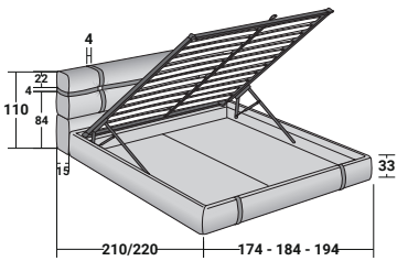
BETTKASTEN-GESTELL FESTE FEDERLEISTEN MIT HÄRTEREGULIERUNG
