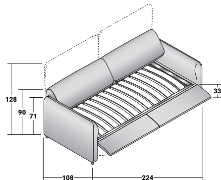
PLANO DE LAMAS AJUSTABLES
