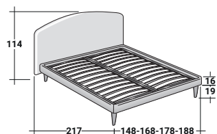
BASE H16 PLANO DE LAMAS AJUSTABLES SOMIER CON MOVIMIENTO ELÉCTRICO
