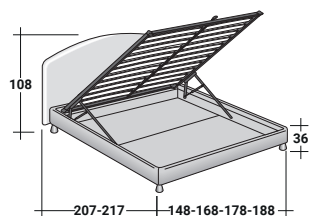
BASE CONTENEDOR PLANO DE LAMAS AJUSTABLES *
