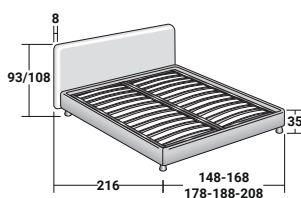
BASE H25 PLANO DE LAMAS AJUSTABLES SOMIER CON MOVIMIENTO ELÉCTRICO
