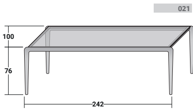
GAUDÌ Table design Matteo Nunziati 2023
